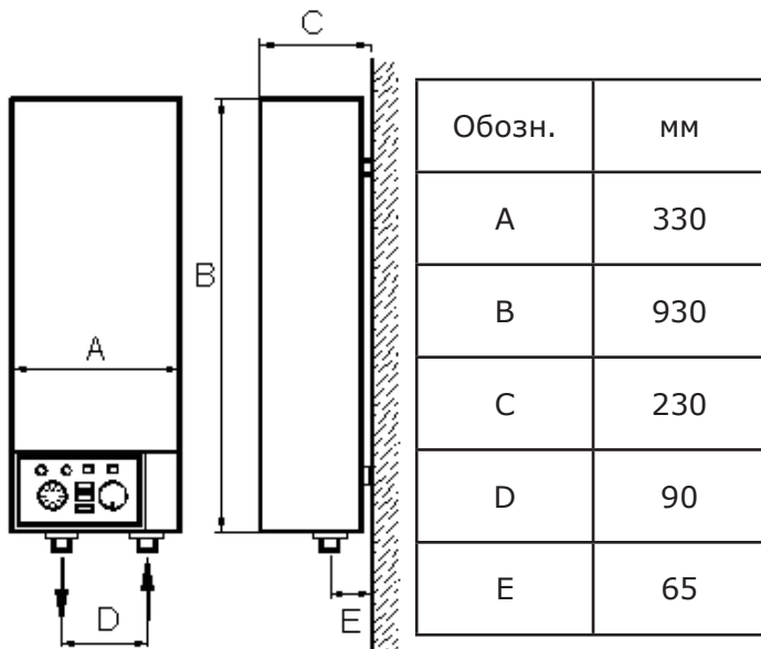
Размеры электрокотла
